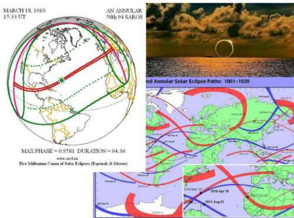
Рисунок №4. Уникальное Библейское солнечное затмение произошло 18 марта 1010 года (An Annular 58th 94 Saros, 15:33 UT).
