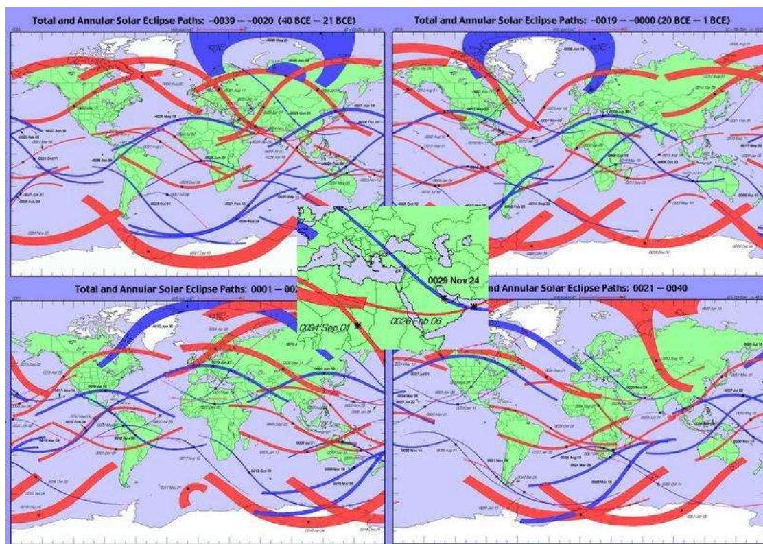
Рисунок №1. Солнечные затмения периода с 40 г. до н. э. по 40 г. В центре находятся затмения примерно в 30-33 годах.
